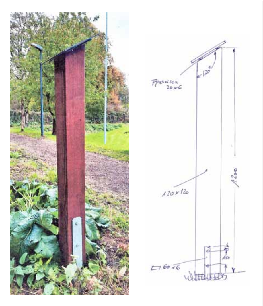
Technische Zeichnung für den Bau einer Stele.
